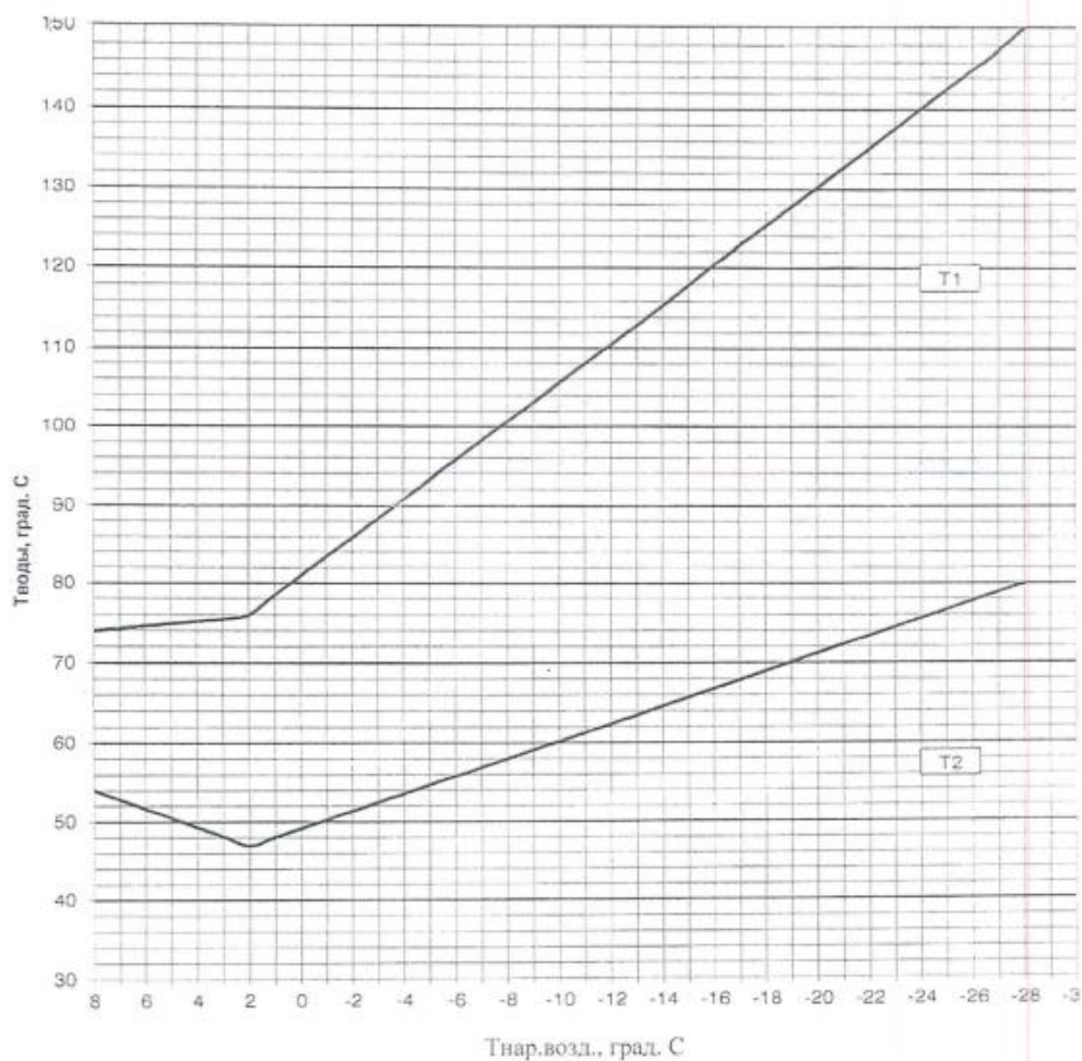
Температурный график отпуска тепловой энергии от Апатитской ТЭЦ на ЦТП г. Кировск на 2024-2025 гг.
