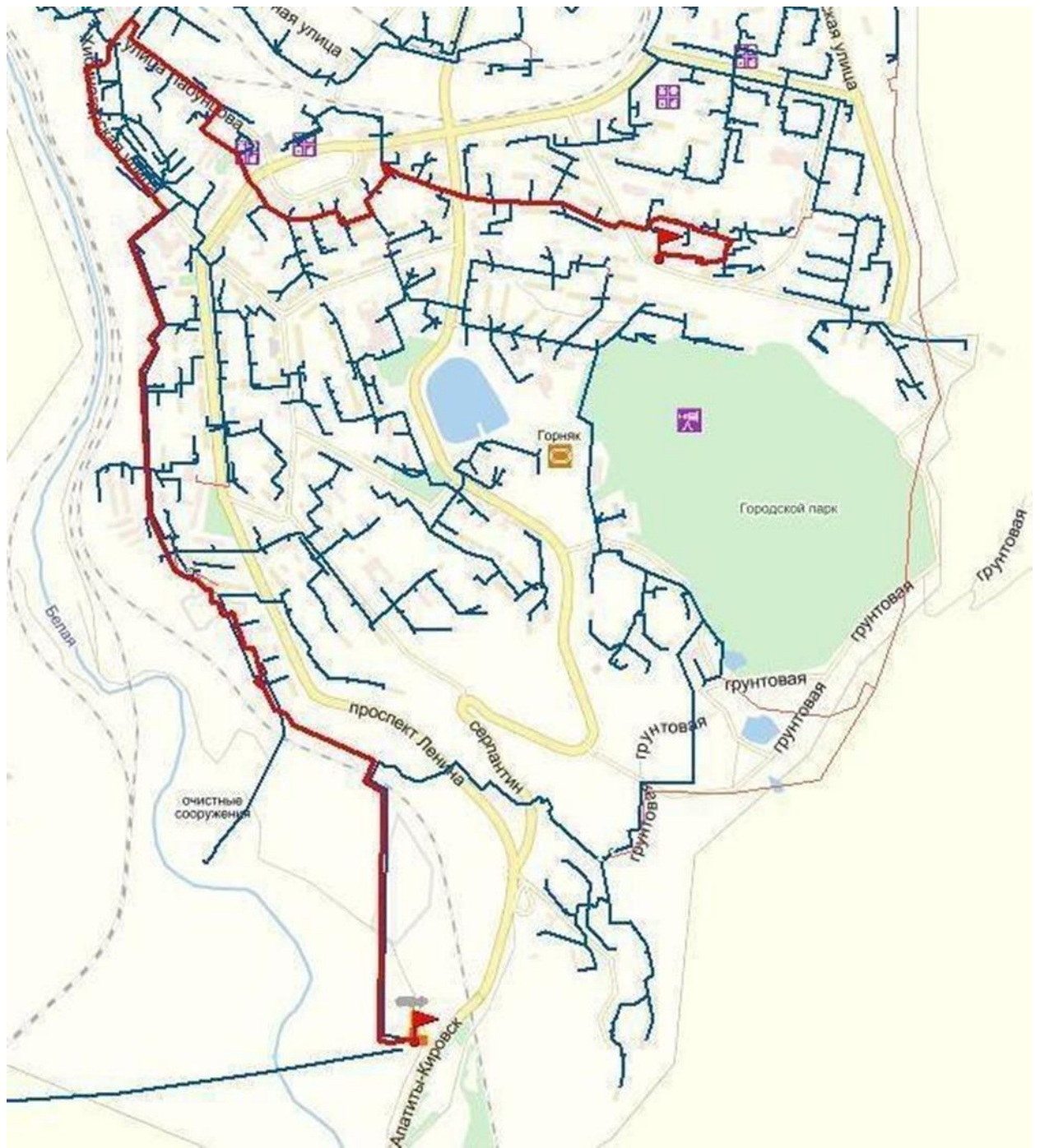
Рисунок 31 - Направление №5 от ЦТП г. Кировска (зона действия АТЭС)
