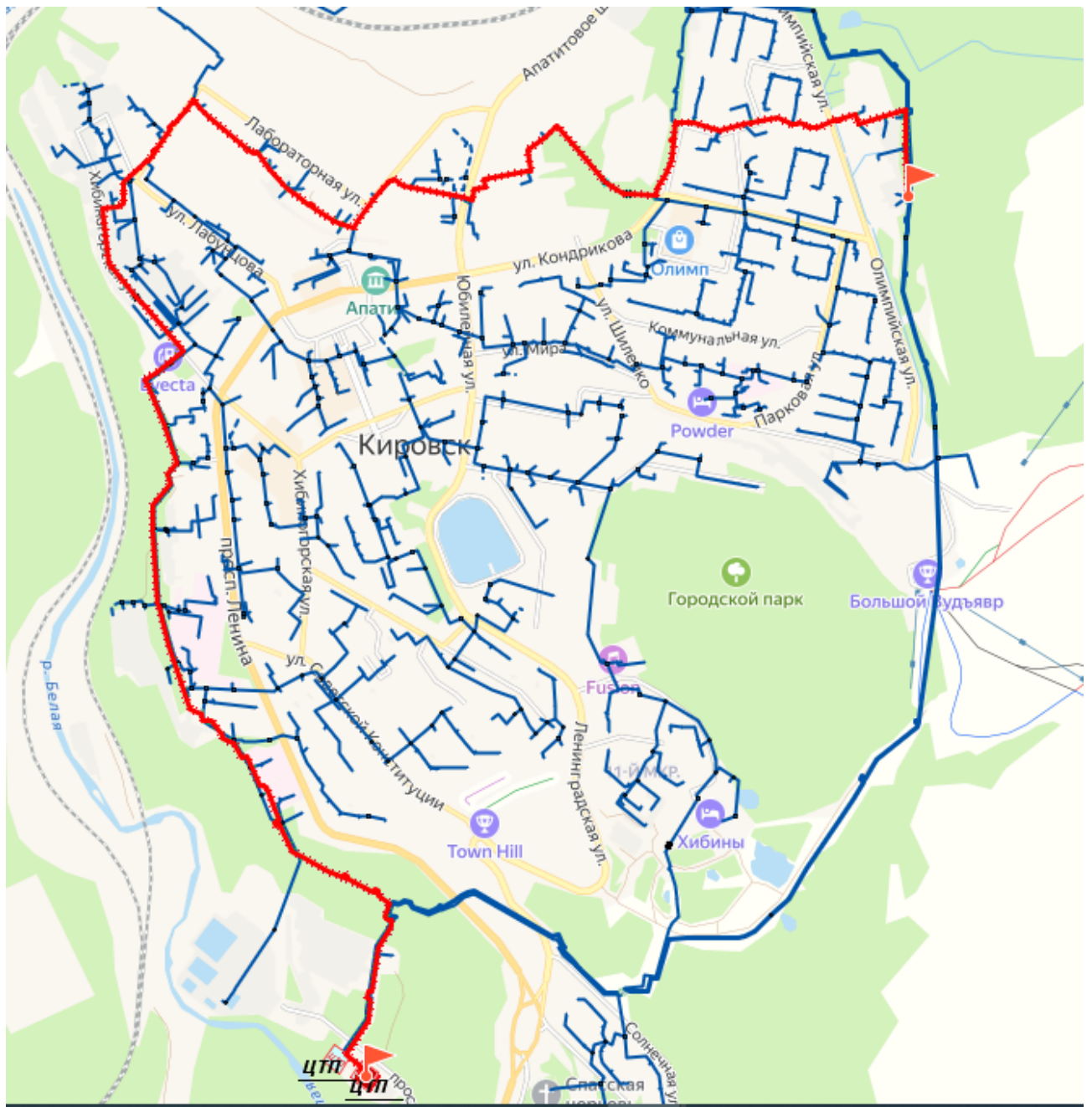
Рисунок 30 - Направление №4 от ЦТП г. Кировска (зона действия АТЭЦ)
