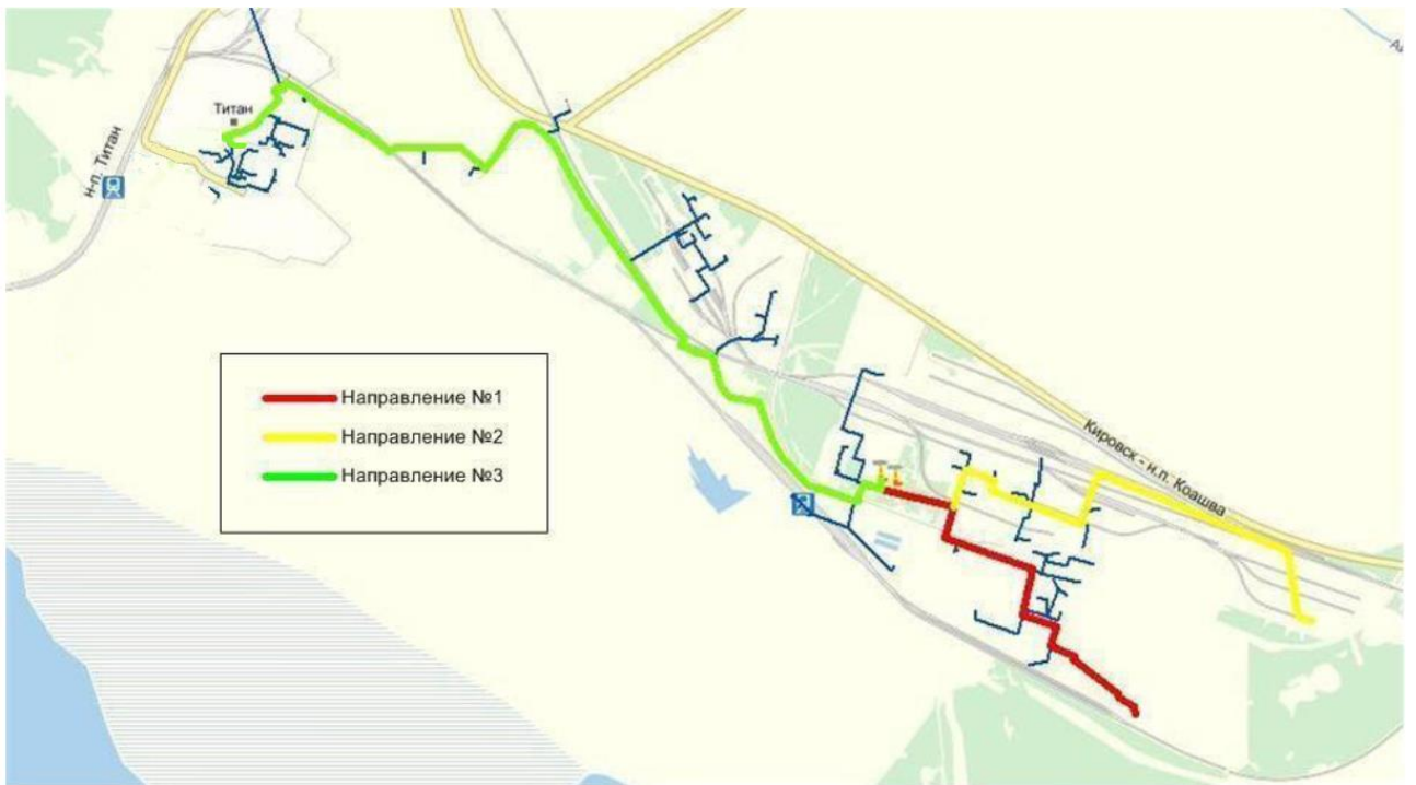
Рисунок 34 - Направления от котельной АНОФ-3
