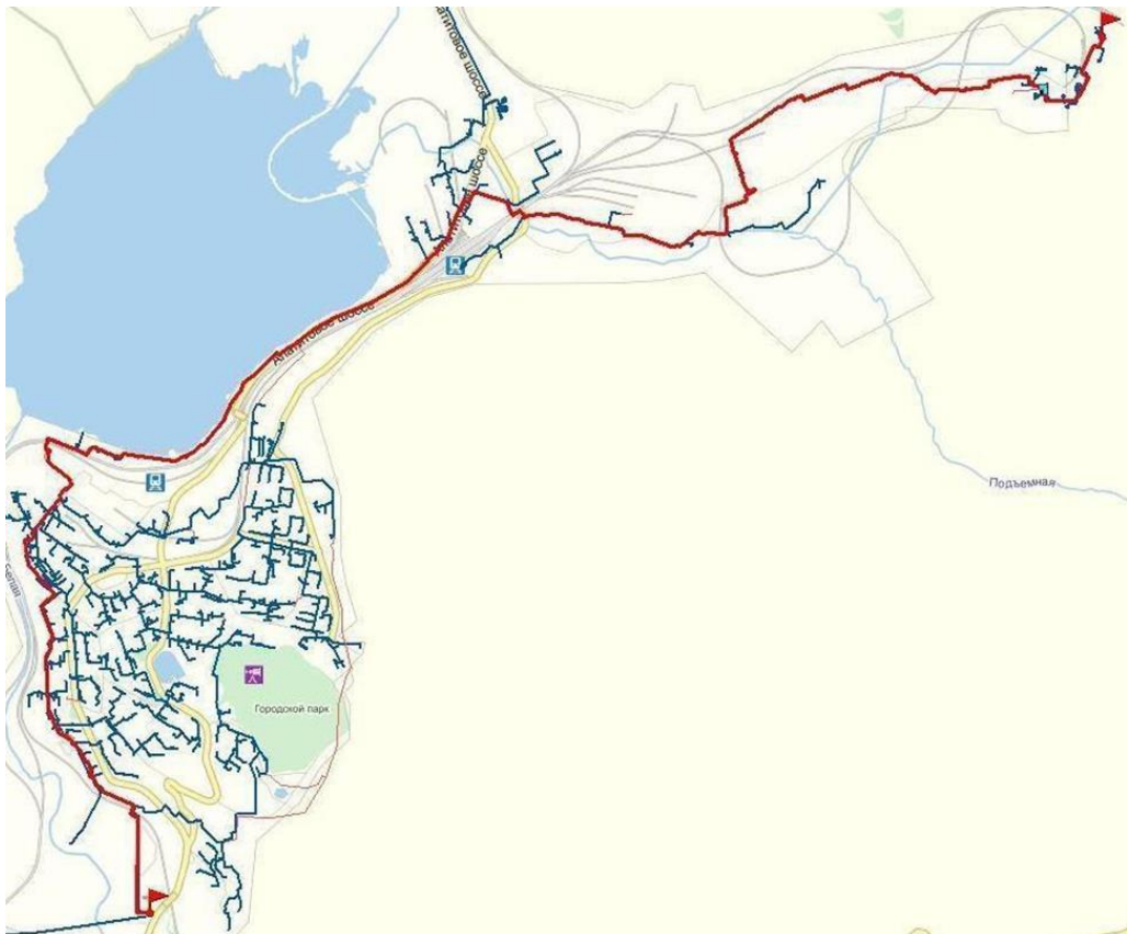
Рисунок 29 - Направление №3 от ЦТП г. Кировска (зона действия АТЭЦ)
