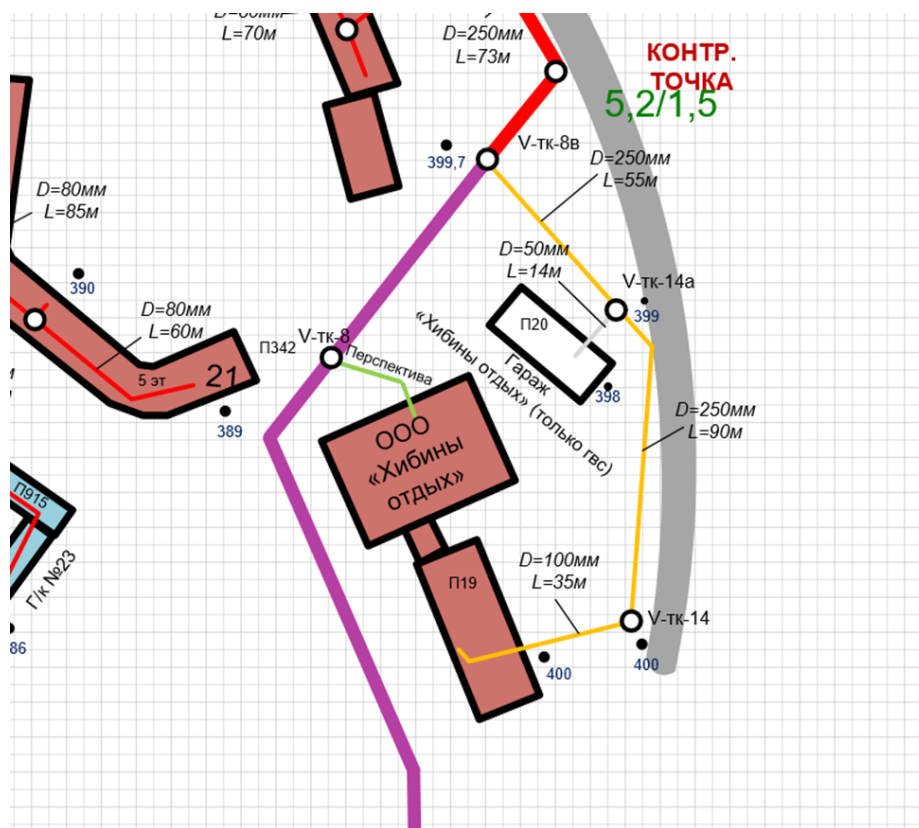
Рисунок 20 - Участок тепловой сети от 5-ТК-8в до 5-ТК-14
