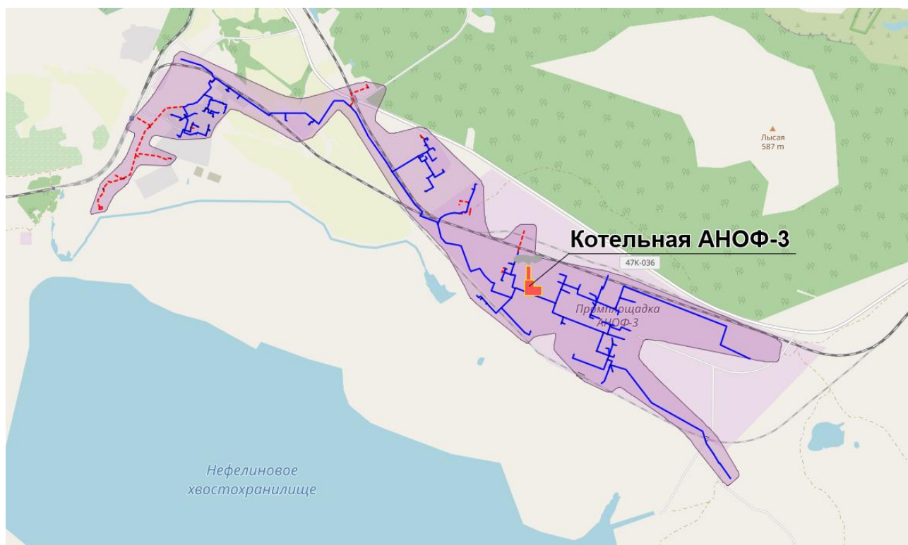
Рисунок 16 – Схема теплоснабжения от котельной АНОФ-3
