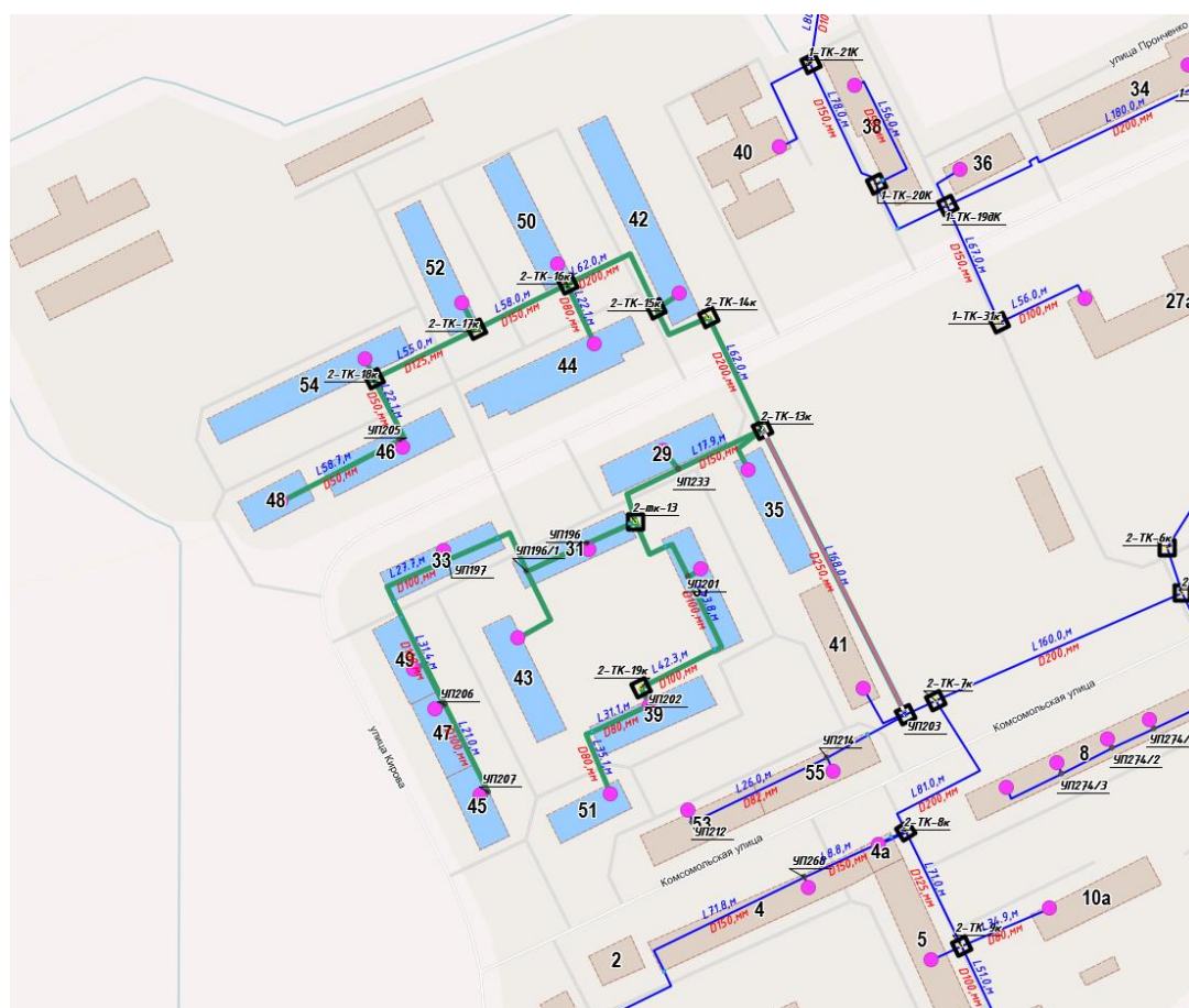
Рисунок 41 - Визуализация отключения запорной арматуры на тепловых сетях от ЦТП г. Кировска
