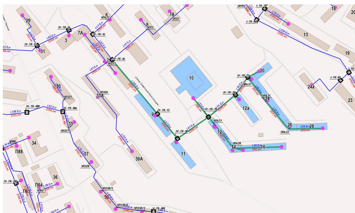
Рисунок 42 - Визуализация отключения запорной арматуры на тепловых сетях от ЦТП г. Кировска
