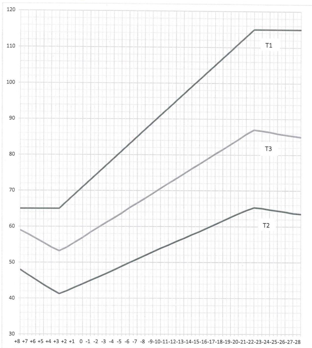
Рисунок 8 - Температурный график отпуска тепловой энергии от ЦТП г. Кировск
